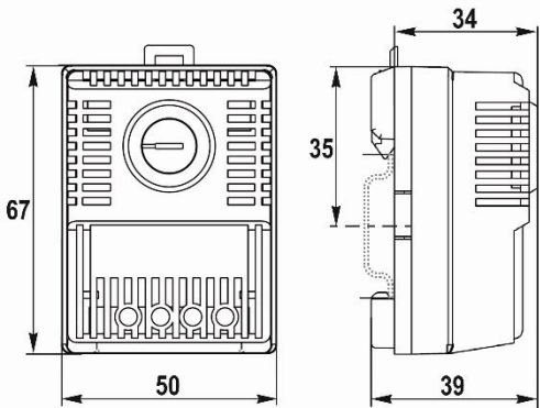
Рис. 1 – Общий вид и габаритные размеры гигростата UNISPLIT 84HF
